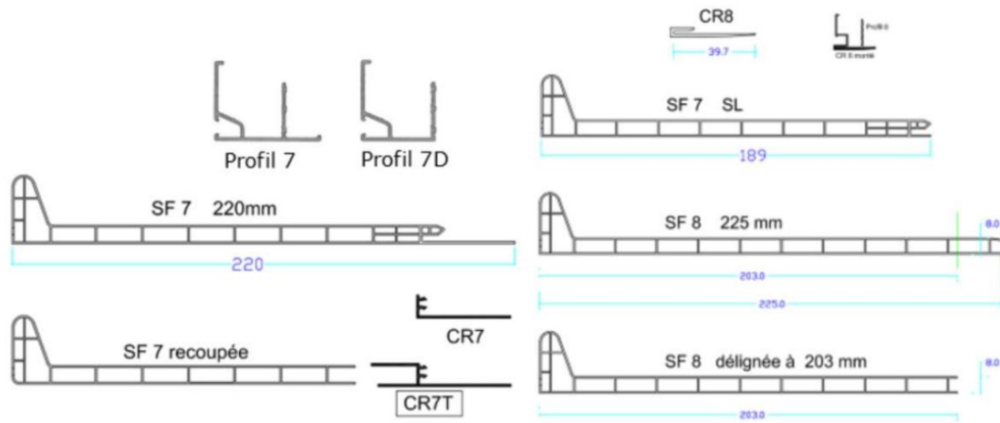
Figure 37 - Sous-faces (SF) et cache-rails (CR)
