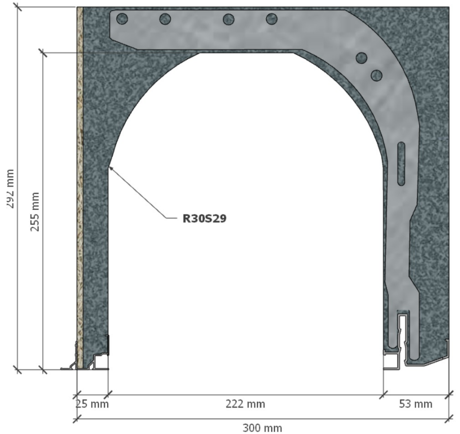
Coffre représenté : C-R30S29 8F-30FR F-NG
