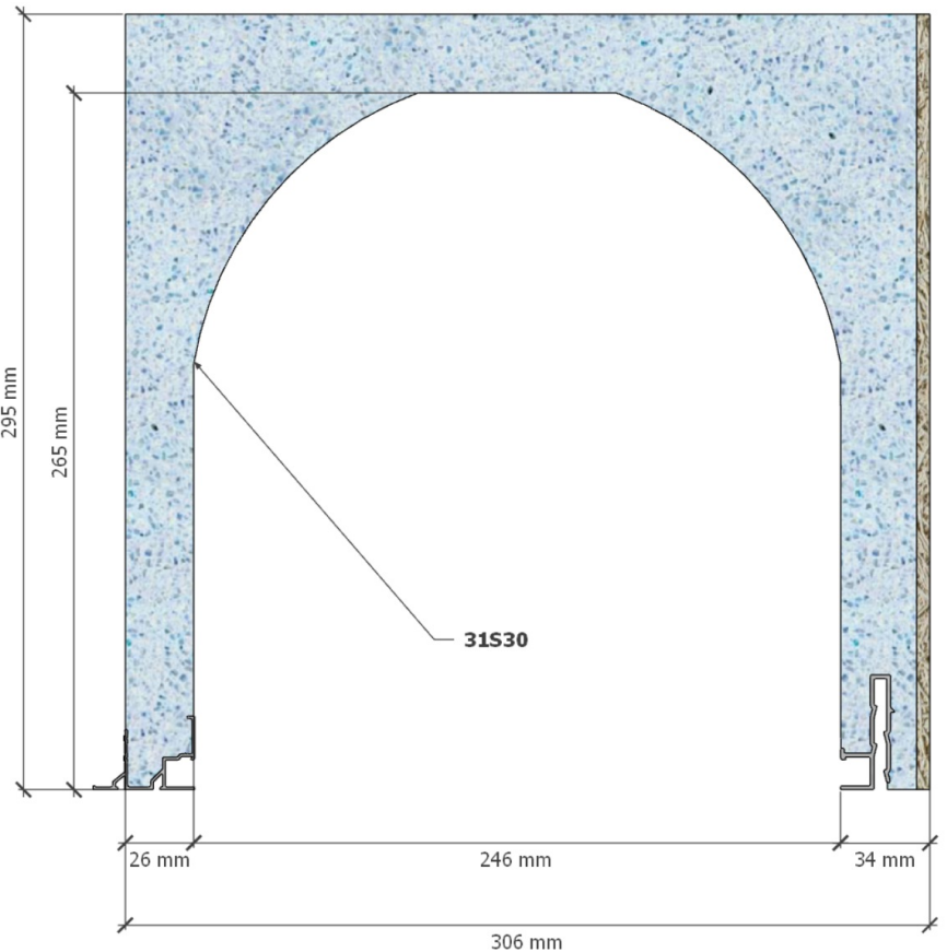
Coffre représenté : C-31S30 8F-8R F
