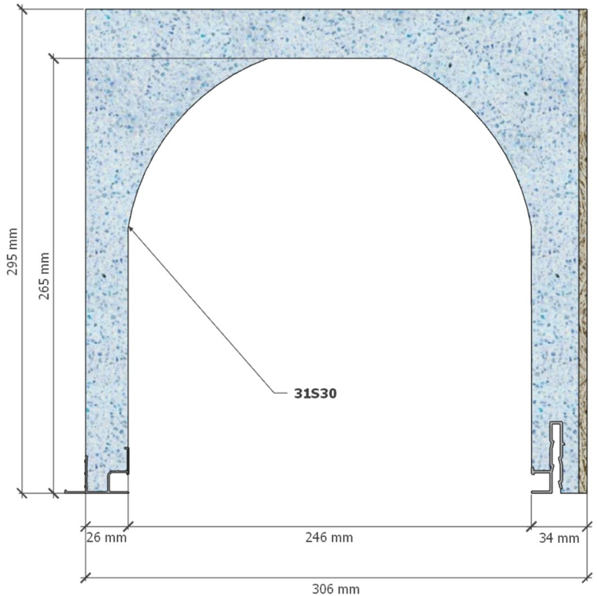
Coffre représenté : C-31S30 8-8R F
