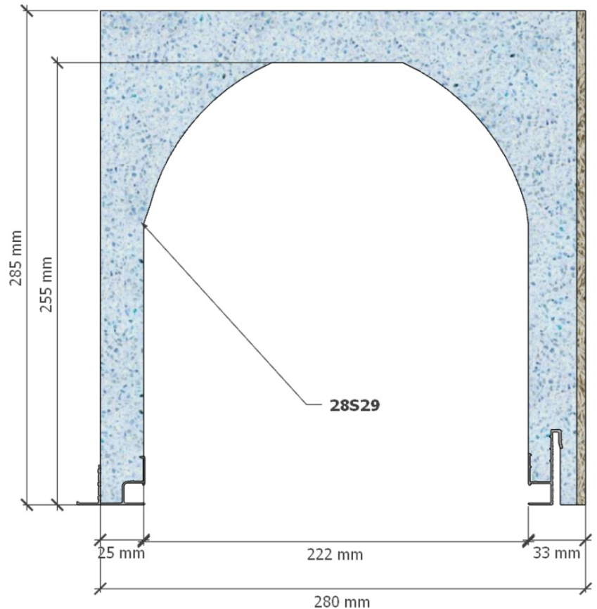
Coffre représenté : C-28S29 8-8E F
