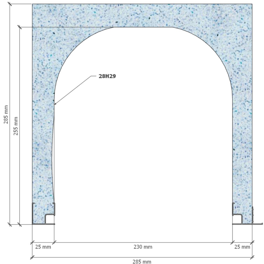
Coffre représenté : C-28H29 8-8R NB
